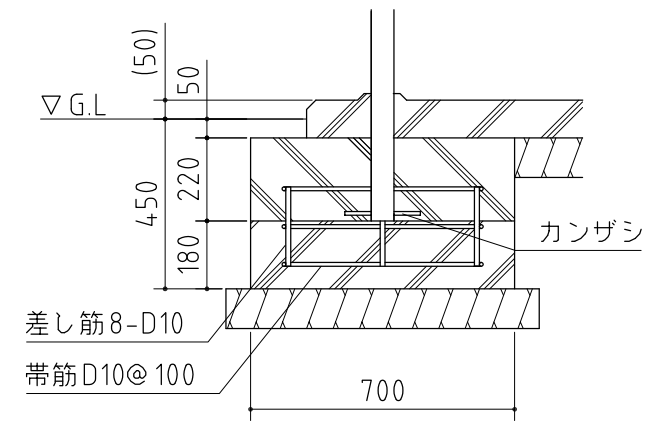
A-A' 断面 1/20
